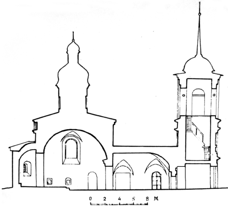
Разрез Мининской церкви по оси восток-запад. Чертеж В. А. Лебедевой, 1960-е гг.
